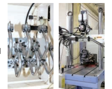
▲脉冲试验机 ▲振动试验
