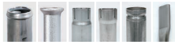
▲膨胀节加工 ▲喇叭口加工 ▲缩管加工 ▲扩管加工 ▲强力旋压加工 ▲压扁加工
