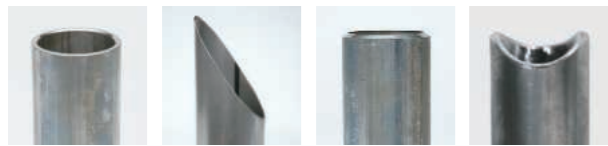
▲直角切割 ▲斜角切割 ▲破口加工 ▲鞍型加工
